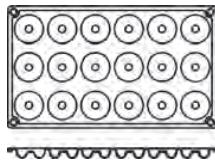
FR005 MINI SAVARIN mm Ø 41 x 12 H vol. 12 ml 18 impronte/indents
