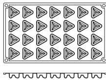
FR076 MICRO SAVARIN TRIANGOLO mm 30 x 30 x 13,5 H vol. 6,5 ml 28 impronte/indents
